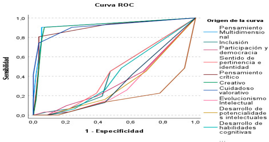
Figura 2 2. Curva ROC
